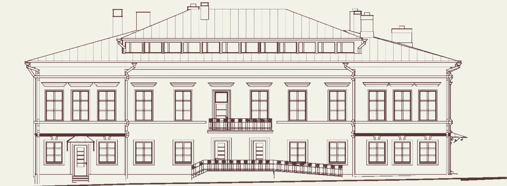
JULKISIVU LÄNTEEN
